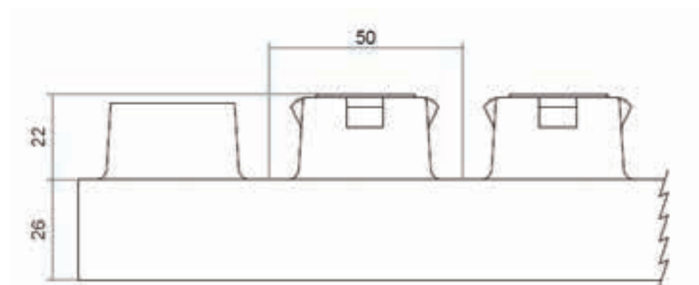
Detalle del perfil (cotas en mm)
