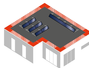
Sistema de fijación cubierta plana. Comprobar separación de baterías según latitud del lugar e inclinación elegida.
